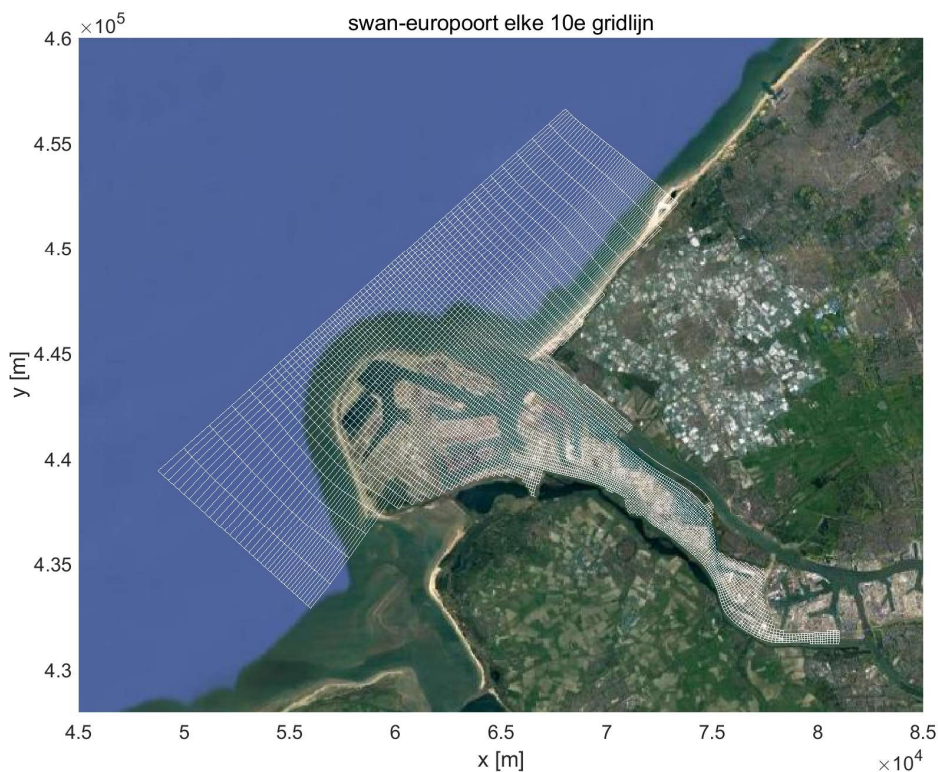
Figuur 1 Rekenrooster swan-europoort (elke 10e roosterlijn van het rekenrooster is zichtbaar)
