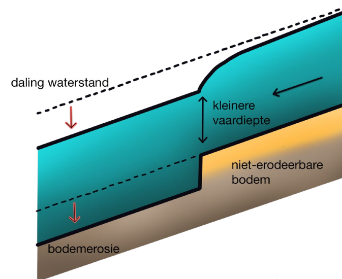
Figuur 5b. Vermindering van de vaardiepte boven vaste lagen als gevolg van bodemerrosie.
