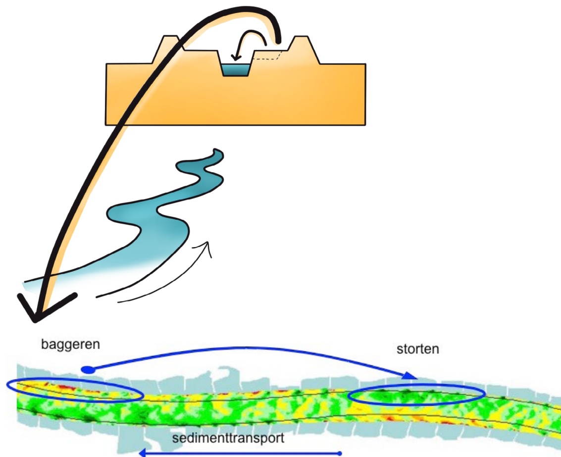
Figuur 12. Sedimentbeheer in de Waal: het zand dat op ondieptes wordt weggebaggerd wordt bovenstrooms in diepe buitenbochten teruggestort. Het zand zal door de rivier weer naar de ondieptes worden verplaatst waarna de stap van baggeren en terugstorten wordt herhaald.
