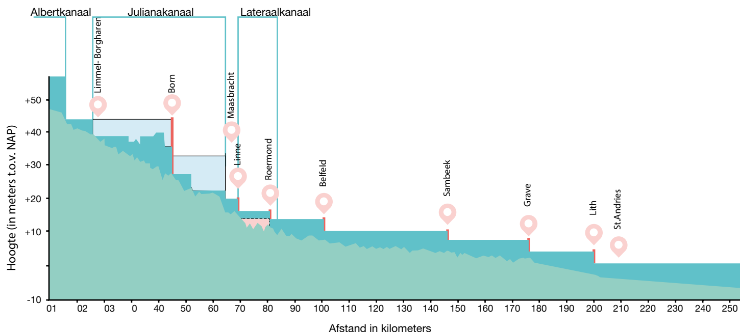
Figuur 8. Langsprofiel van de Maas in Nederland. De rivier is voor een groot deel gestuwd (rode lijnen zijn stuwen) en daardoor is deze rivier morfologisch weinig actief. Dit geldt ook voor de Nederrijn-Lek.
