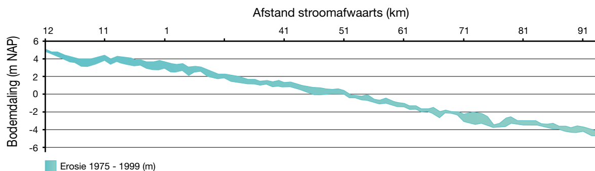
Figuur 5a. De daling van de bedding van de Bovenrijn en Waal tussen 1975 (bovenste lijn) en 2000 (onderste lijn). Harde lagen zijn relatief hoog komen te liggen en vormen een soort drempels voor de scheepvaart, met geringe aflaaddieptes tot gevolg.
