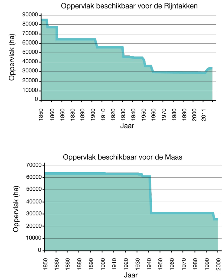
Figuur 4. De verandering in de beschikbare oppervlakte voor de Rijntakken (boven) en de Maas (onder) sinds 1850.
