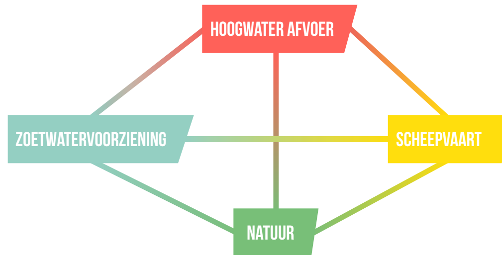
Figuur 10. De verschillende functies van de rivier hebben soms onderling strijdige wensen of stellen tegenstrijdige eisen
