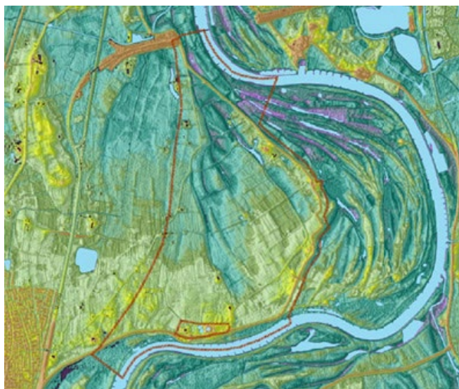
Figuur 11. Kronkelwaarden (zandruggen) langs de IJssel, ontstaan in het verleden en nu onderdeel van een 'gestold' rivierenlandschap.
