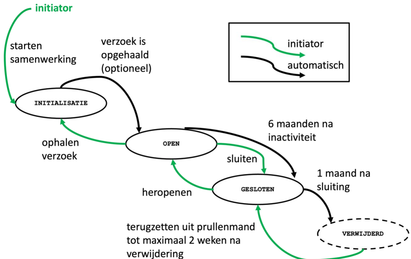
Figuur 3: Toestandsdiagram samenwerkingen (SWF-API v5)
