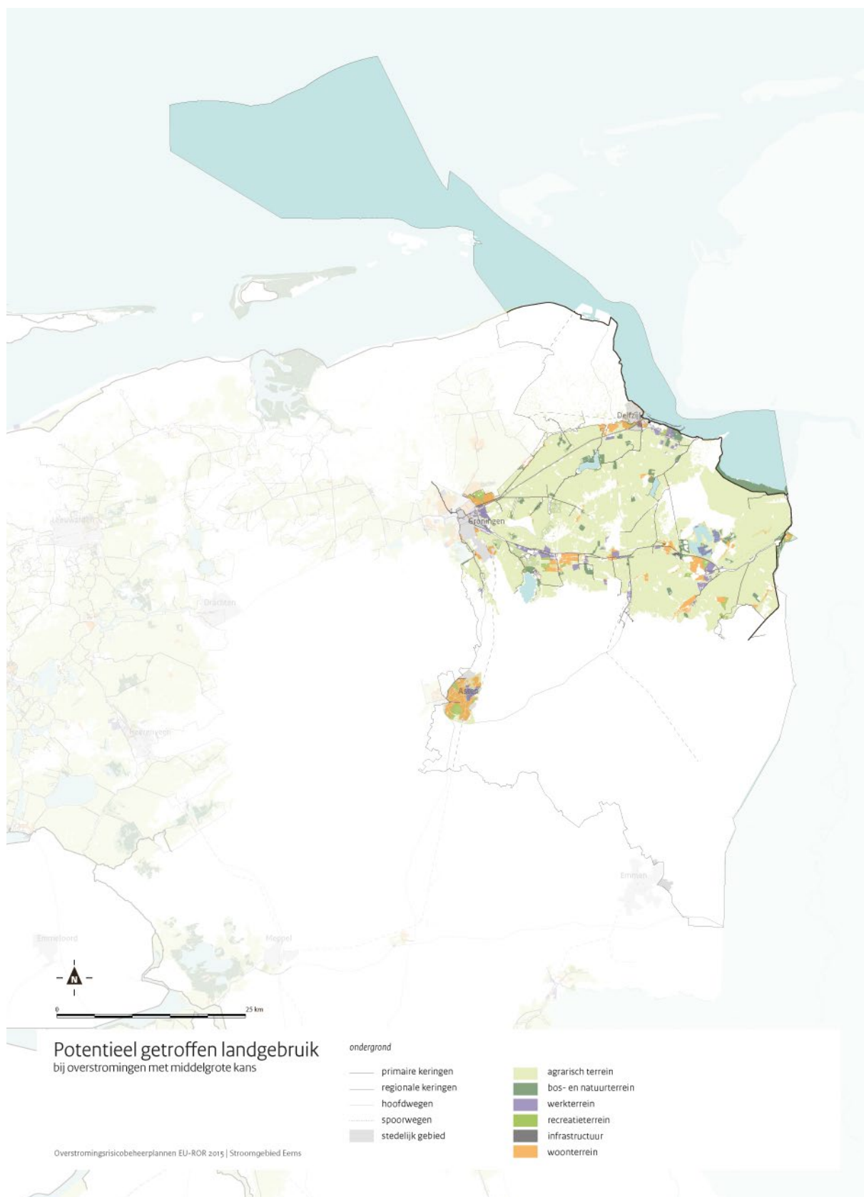
Kaart 13 Potentieel getroffen landgebruik bij overstromingen met middelgrote kans
