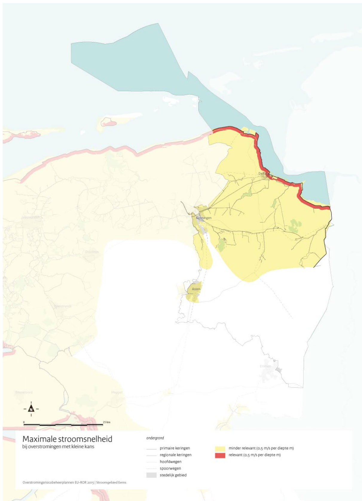
Kaart 26 Maximale stroomsnelheid bij overstromingen met kleine kans
